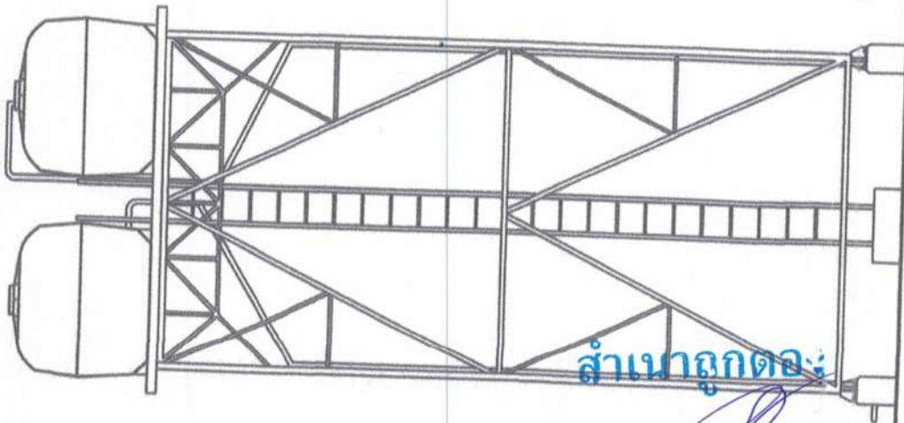
รูปด้าน ขนาด 1:50
