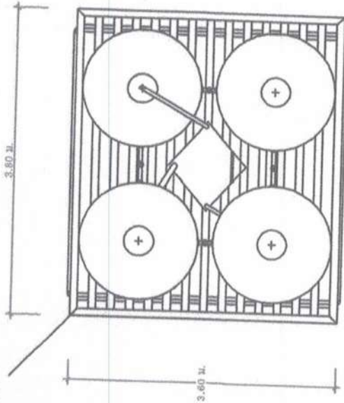
แปลนโครงสร้างเหล็กกับถังน้ำ (แบบใหม่) ขนาด 3.60 x 3.60
