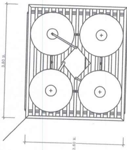
แปลนโครงสร้างเหล็กกับถังน้ำ (แบบใหม่)
